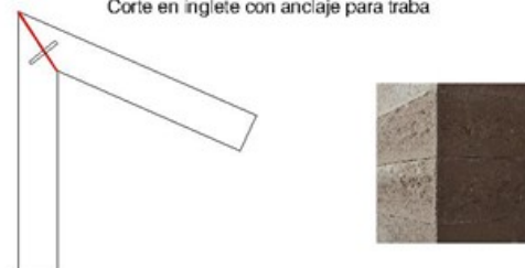
Corte en inglete con anclaje para traba
