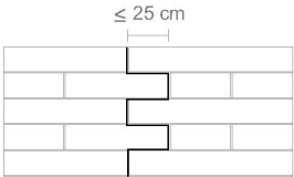
Junta contracción-dilatación dentada Contraction-dilation joint toothed
